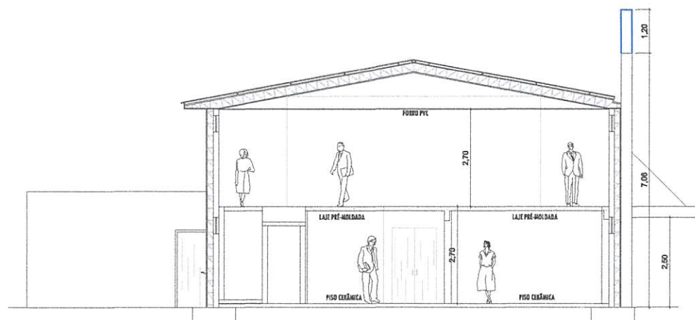
CORTE B ESCALA 1:100
