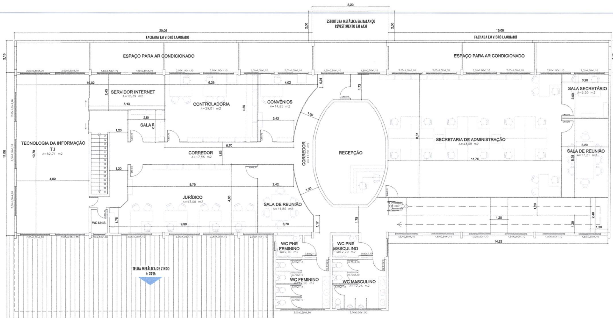
PLANTA BAIXA - PAV. SUPERIOR ESCALA 1:100
